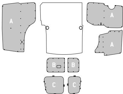
Modelo - Model L1 H1
